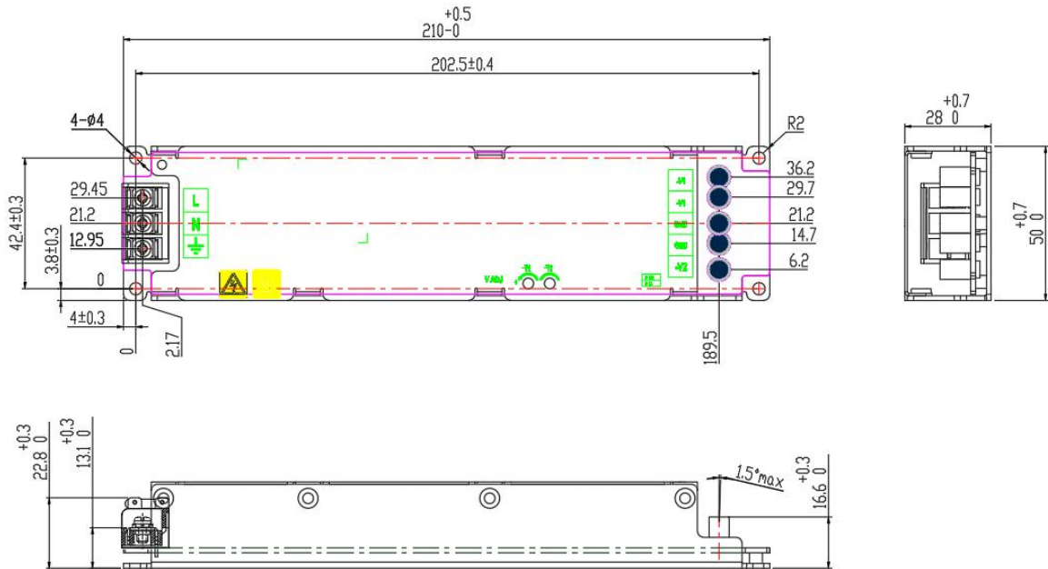
外形尺寸及安装孔——端子坐标图
